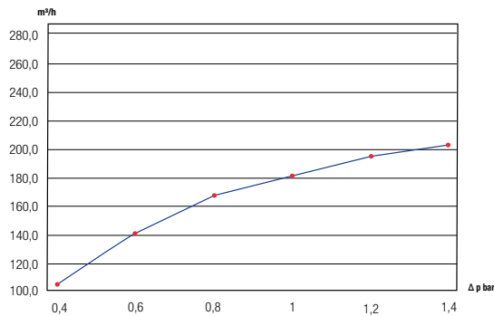
DN100 - 1xA
